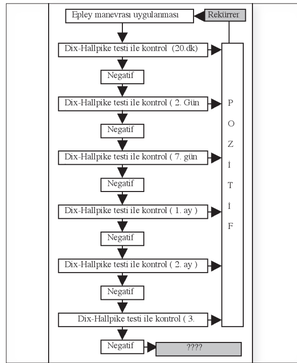
Resim 1. Çalışmanın algoritması
